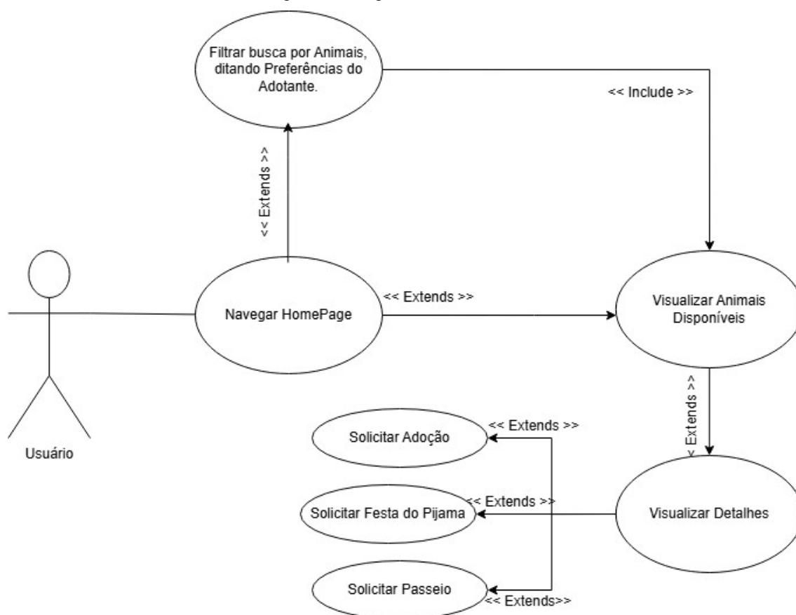
Figura 05: Diagrama de caso de uso
