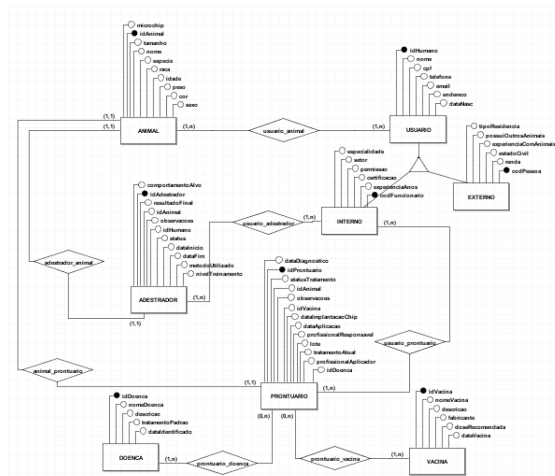
Figura 06: Modelagem de banco de dados conceitual
