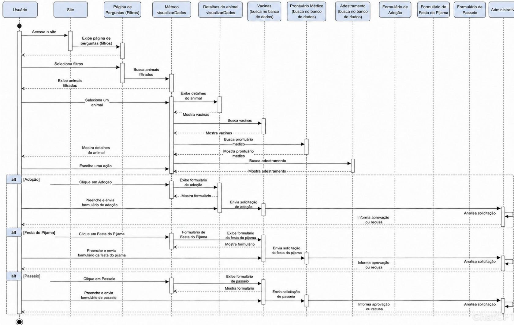
Diagrama de Sequência - Sistema de Adoção de Animais
