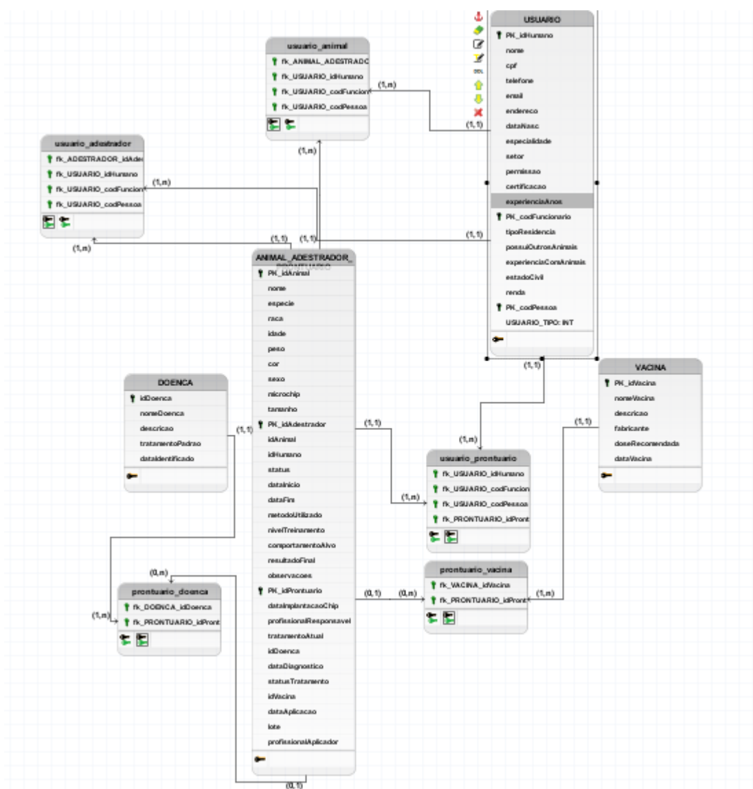
Figura 07: Modelagem de banco de dados lógico
