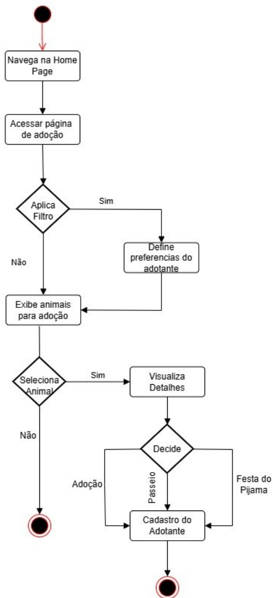
Figura 09: Diagrama de atividades
