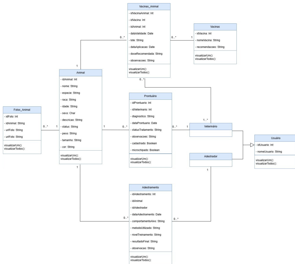
Figura 08: Diagrama de classe
